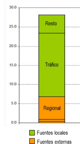
Contribuciones a la media anual de \text{NO}_2 ( \mu\text{g}/\text{m}^3 )
